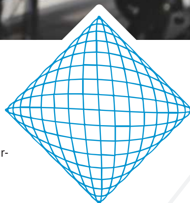
Lissajous Figur
